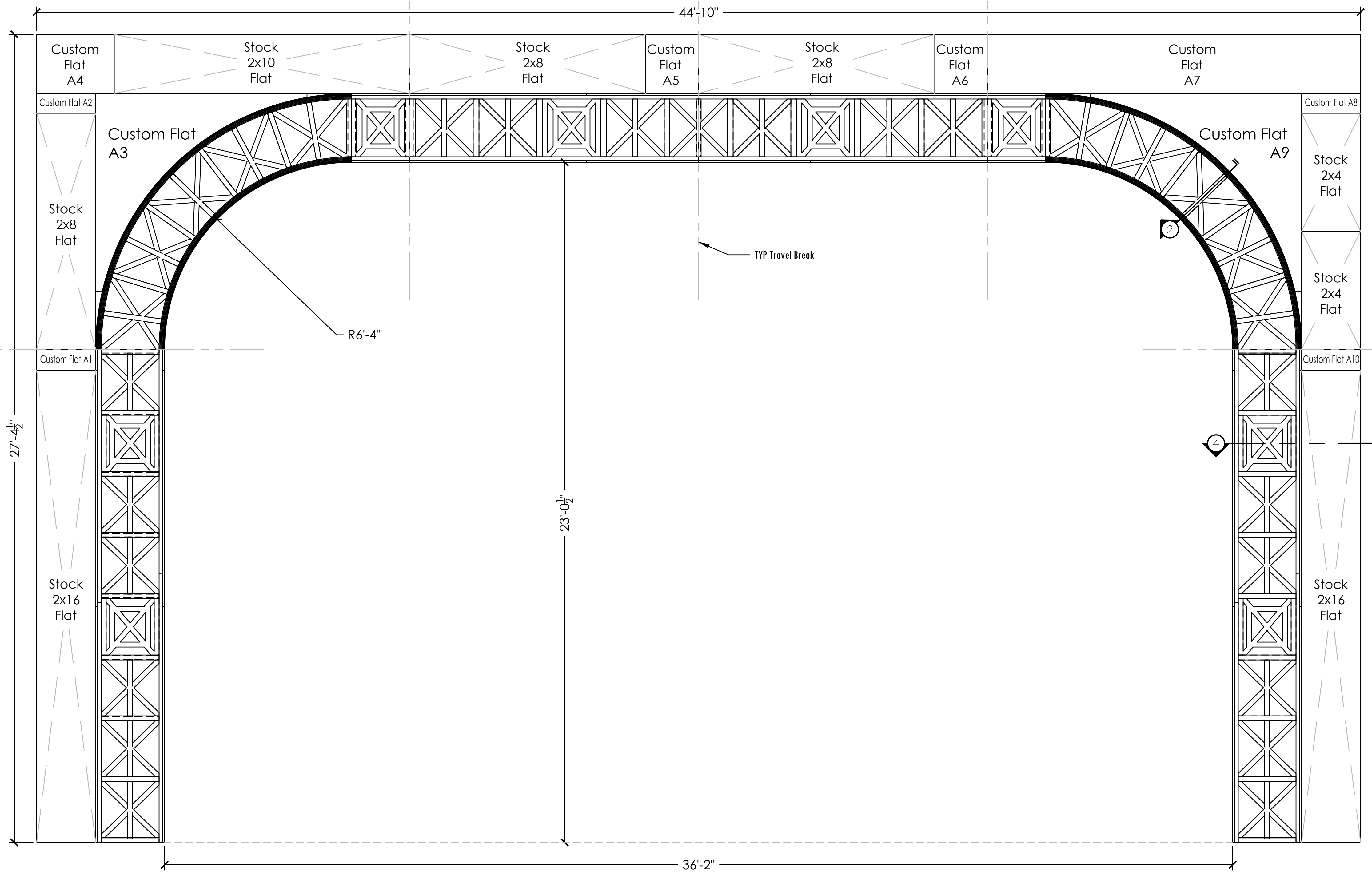
1 D.S. Portal Front View Scale: 1/2"=1'-0"
